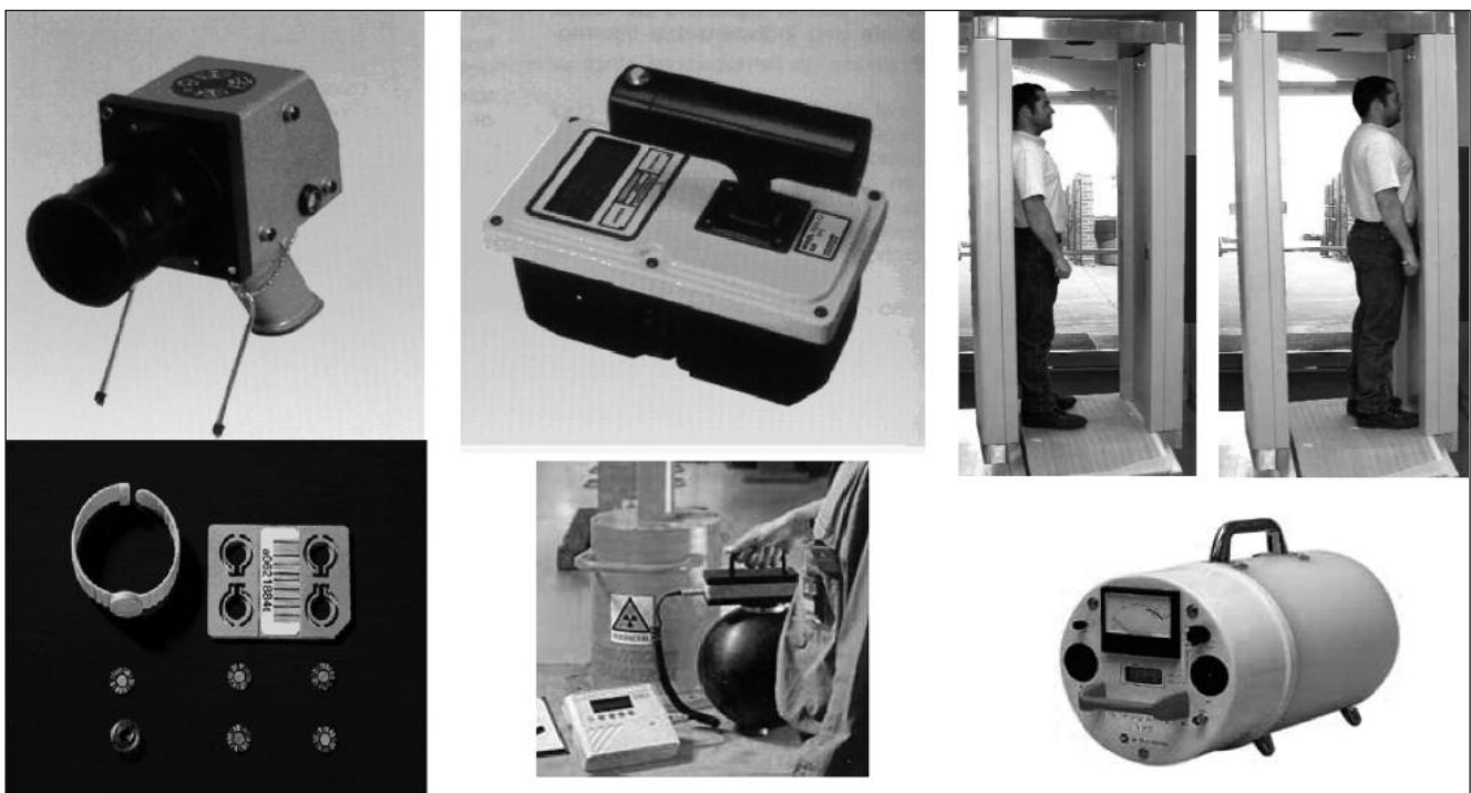
FIGURA 2. Sistemas de detección de la radiación habituales en protección radiológica: cámara de ionización; detector Geiger; monitor de contaminación, de centelleo; dosímetros termoluminiscentes; monitores de neutrones.
