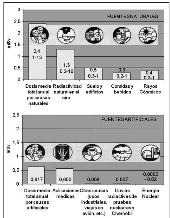
FIGURA 5. Contribución de las diferentes fuentes de radiación naturales y artificiales a la dosis media total anual recibida por la población mundial 3 .
