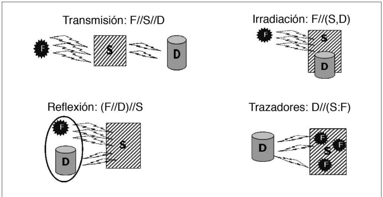
FIGURA 3. Clasificación de los tipos de aplicaciones de las radiaciones ionizantes según la configuración de la fuente (F), el sistema material (S) y el detector (D).
