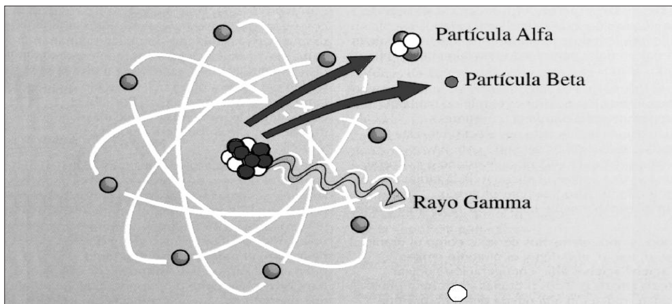
FIGURA 1. Ilustración de los distintos tipos de partículas emitidas por las sustancias radiactivas.
